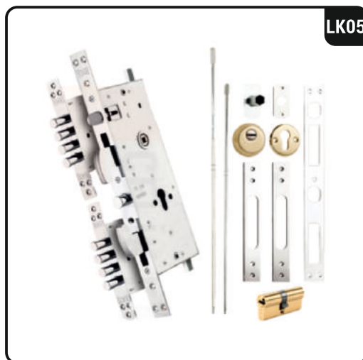
Système de serrure centrale Central Lock System
