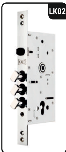
Serrure à Mortaise Avec Pêne Dormant Rotatif Mortise Lock With Rotating Deadbolt
